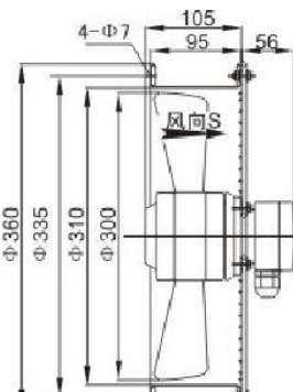
YWF2E300S\ YWF2E300L (185mm אורך הצינור)
