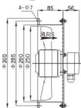
YWF2E250S\ YWF2E250L (175mm אורך הצינור)
