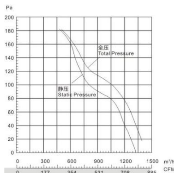
YWF2E250S\ YWF2E250L (175mm אורך הצינור)
